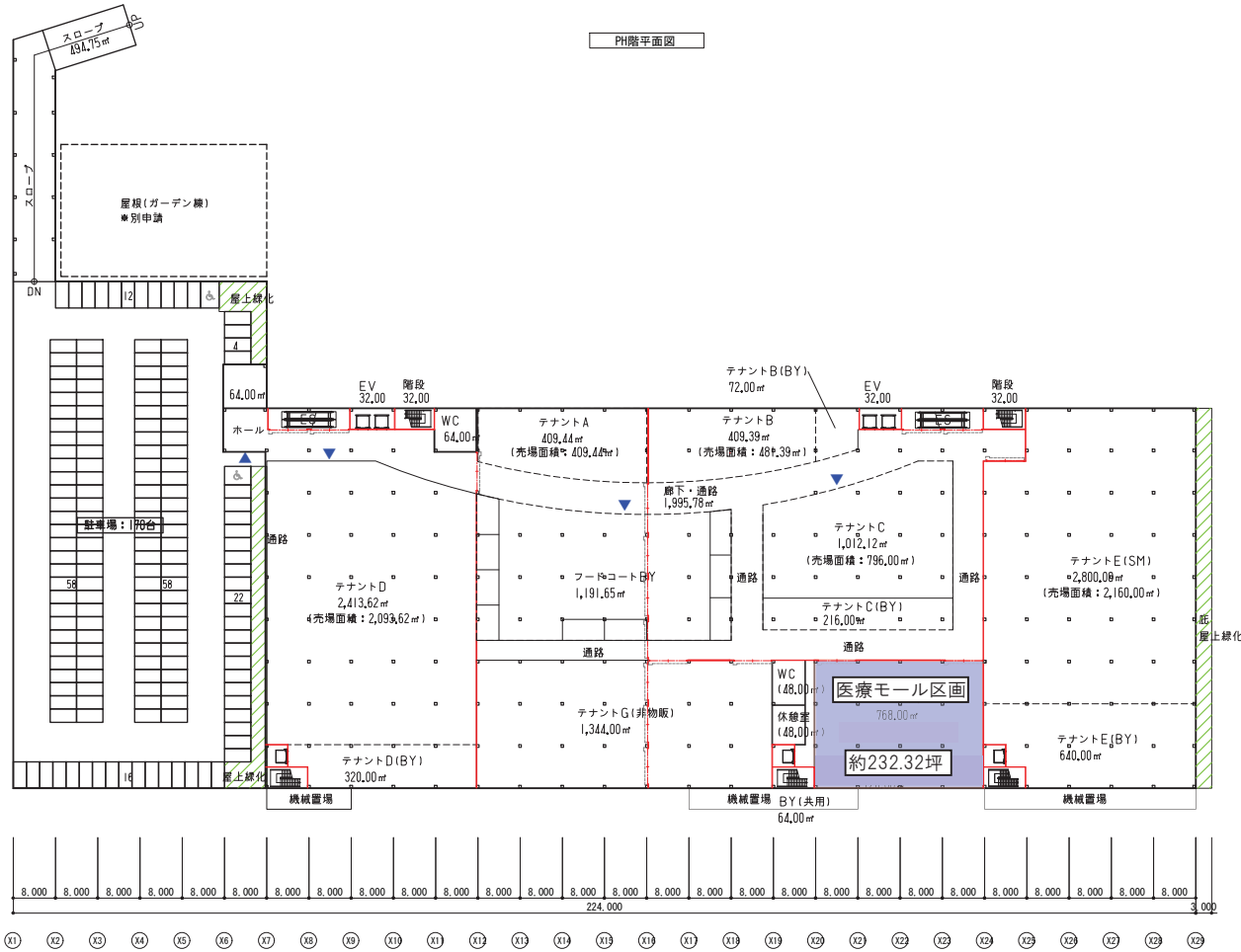
2階平面図
